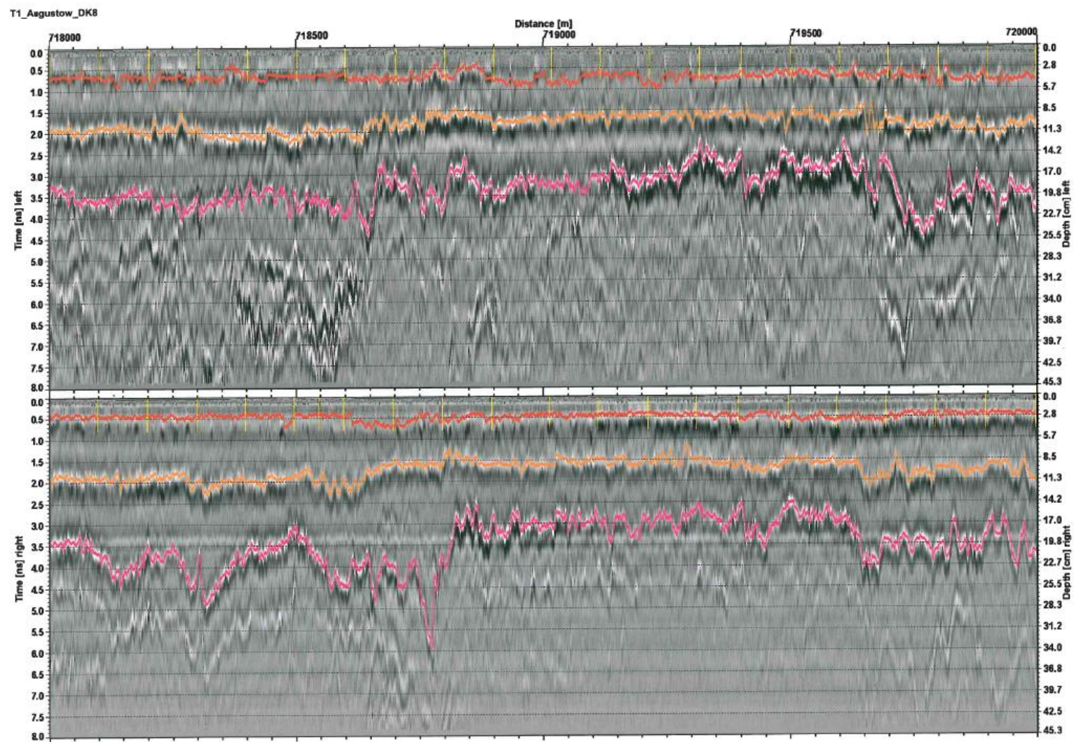
Rysunek 14 Identyfikacja warstw na odcinku 1
