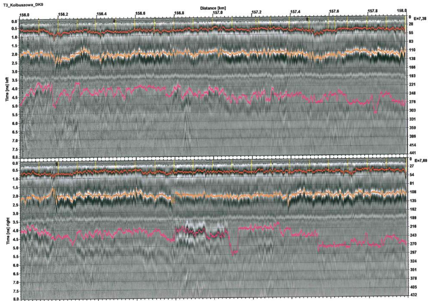
Rysunek 16 Identyfikacja warstw na odcinku 3
