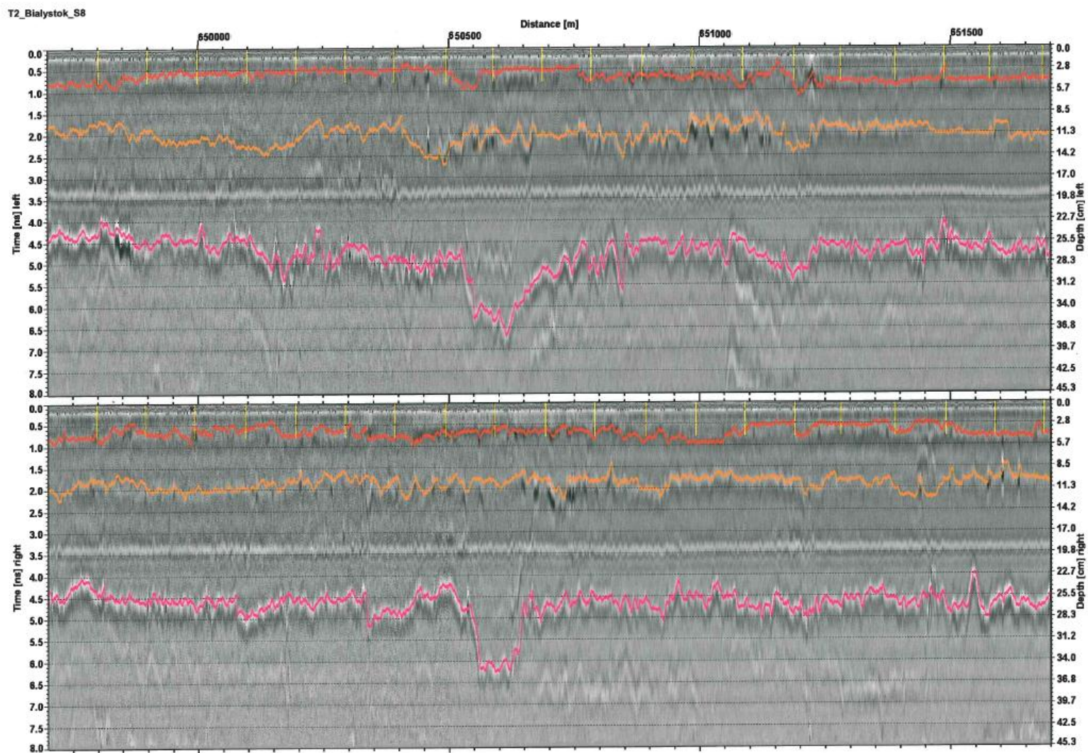
Rysunek 15 Identyfikacja warstw na odcinku 2
