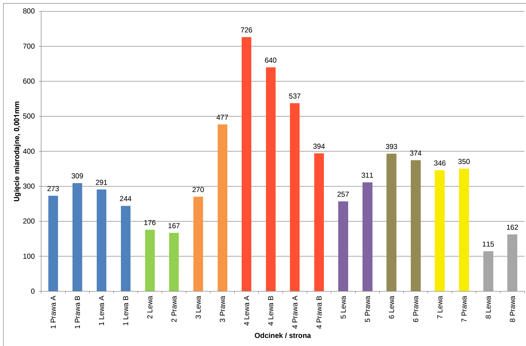
Rysunek 13 Ugięcia miarodajne na poszczególnych odcinkach
