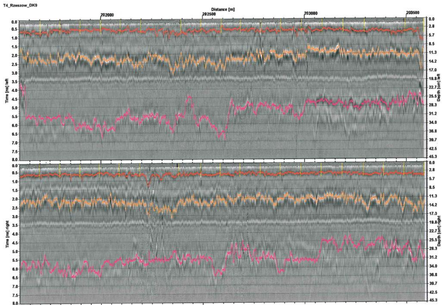
Rysunek 17 Identyfikacja warstw na odcinku 4
