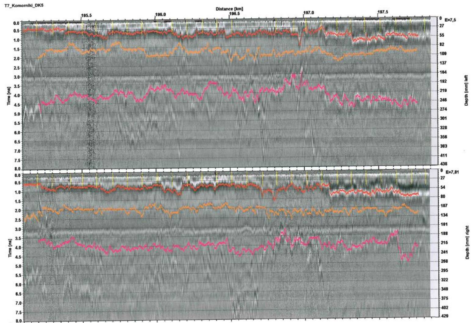
Rysunek 20 Identyfikacja warstw na odcinku 7
