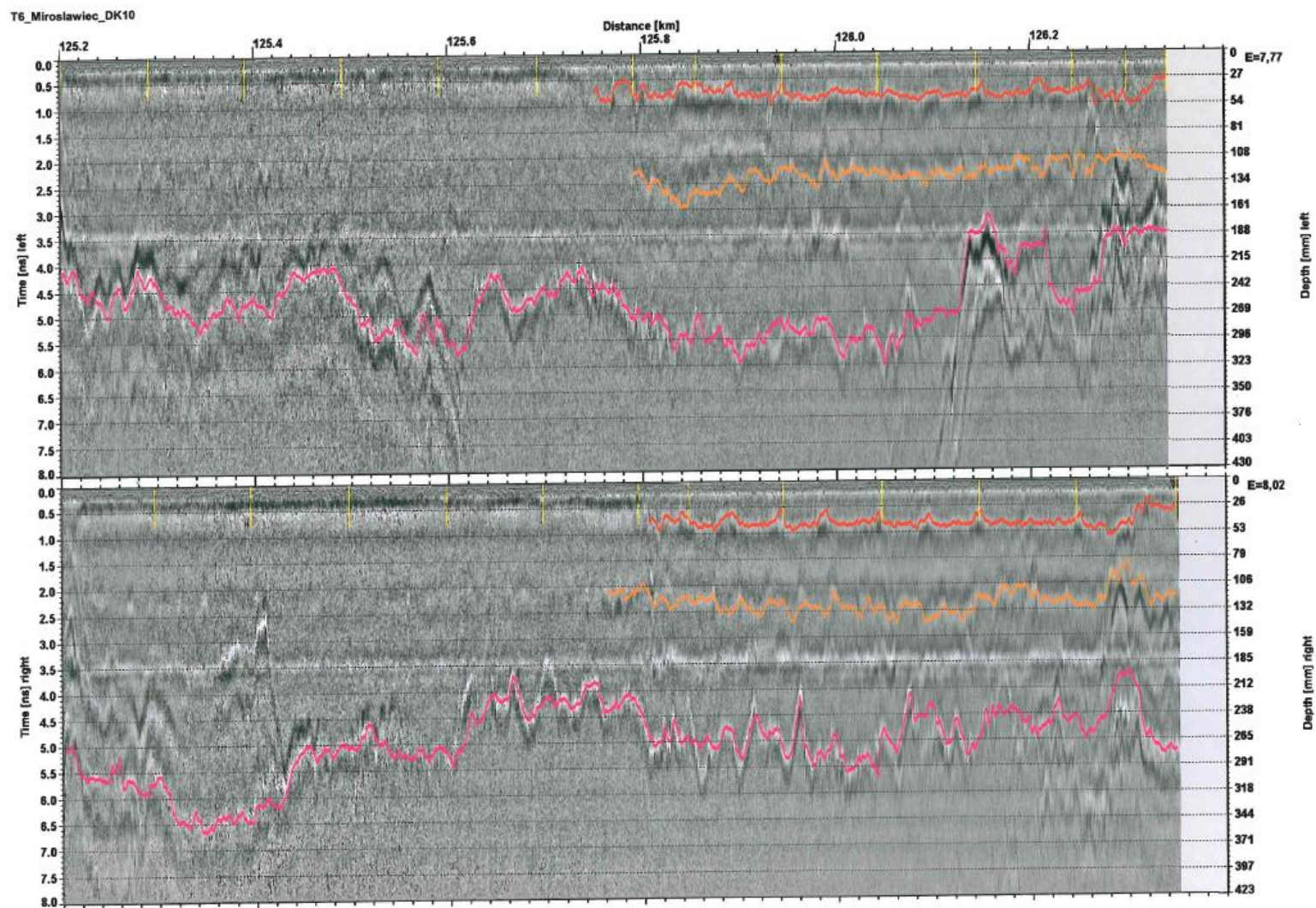
Rysunek 19 Identyfikacja warstw na odcinku 6
