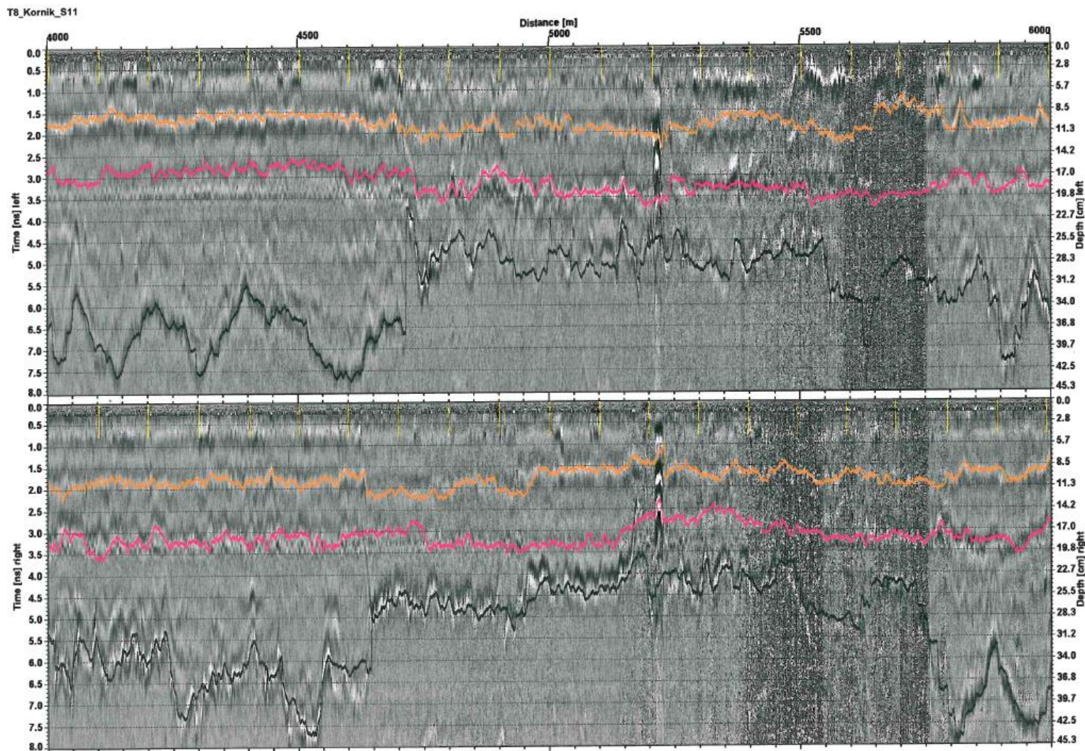
Rysunek 21 Identyfikacja warstw na odcinku 8
